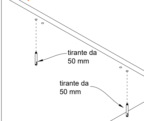
Fig. 2) posizione tiranti da 50 mm nel piano scrivania.
