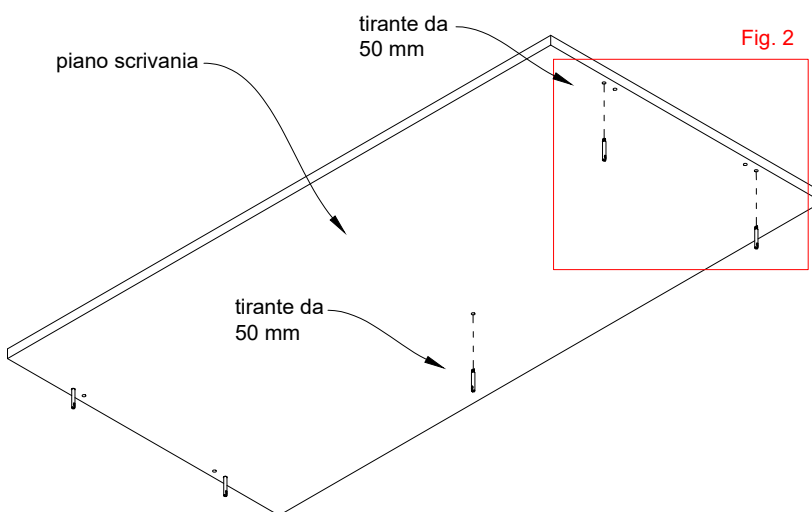
Fig. 2) posizione tiranti da 50 mm nel piano scrivania.
