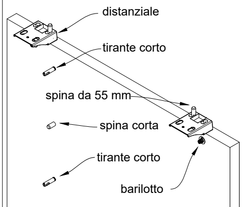
Fig. 2) posizione tiranti da 50 mm nel piano scrivania.
